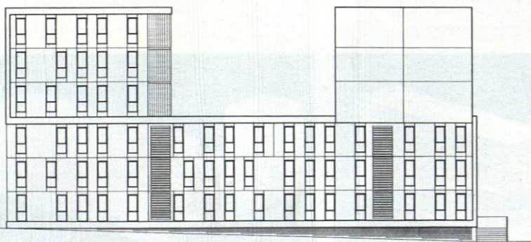
07 - ALZADO OESTE
